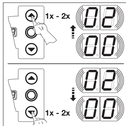
Ill. 6-49: Sélection du numéro de fonction
