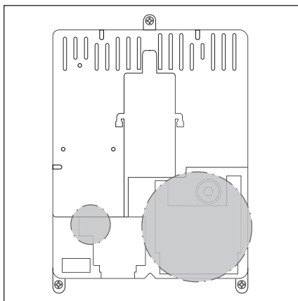
III. 4-17: Position des raccords de câble d'alimentation X10 et X59 sur la platine de commande
