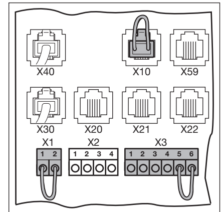
III. 4-31: Ponts enfichables X1/X3, prise pontée X10
