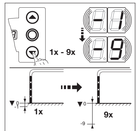
III. 6-31: Réglage de la fin de course Fermé en avançant dans le sens Fermé
