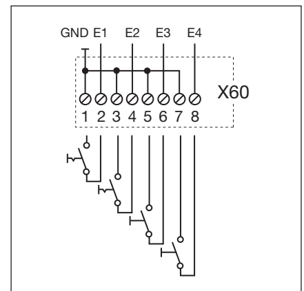
III. 7-17: Raccordement des entrées E1 à E4
