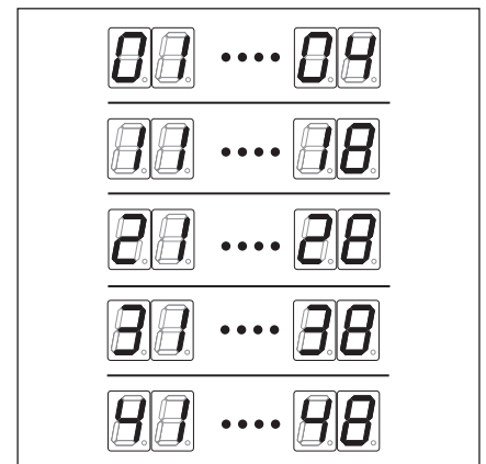
III. 8-15: Affichage des numéros d'erreur 0 1... 04 à 4 1... 48
