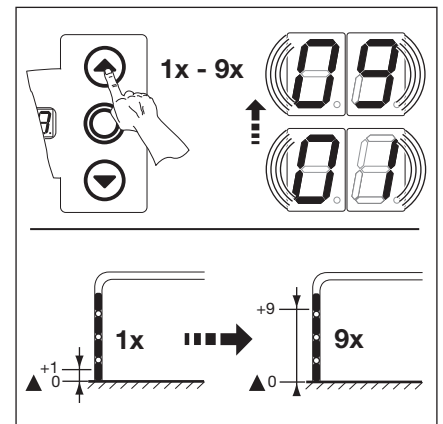
III. 6-30: Réglage de la fin de course Fermé en reculant dans le sens Ouvert
