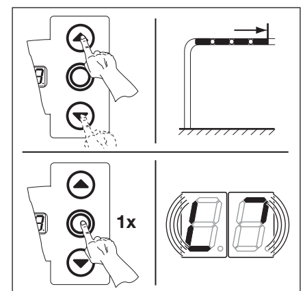
Ill. 6-22: Programmation de la fin de course Ouvert
