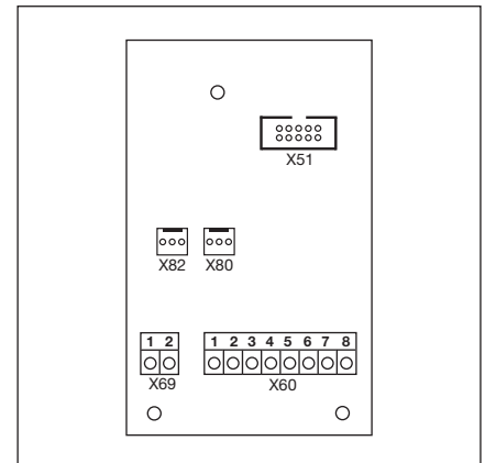
III. 7-15: Conception de la platine
